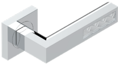
Poignée de porte - Carré de 7 & 8 mm Insert cristal LALIQUE Door handle - 7 & 8 mm spindle LALIQUE crystal insert La paire / the pair : B8C.DHSC1 L'unité / the unit : B8C.DHSC1/S
